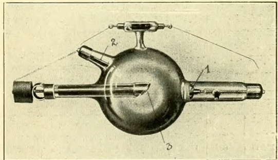
רענטגען-טרייבל (מיט לופט-קילונג): (1 קאַטאָד, 2 אַנאָד, 3 לופט-געקילטער אַנטי-קאַטאָד.
